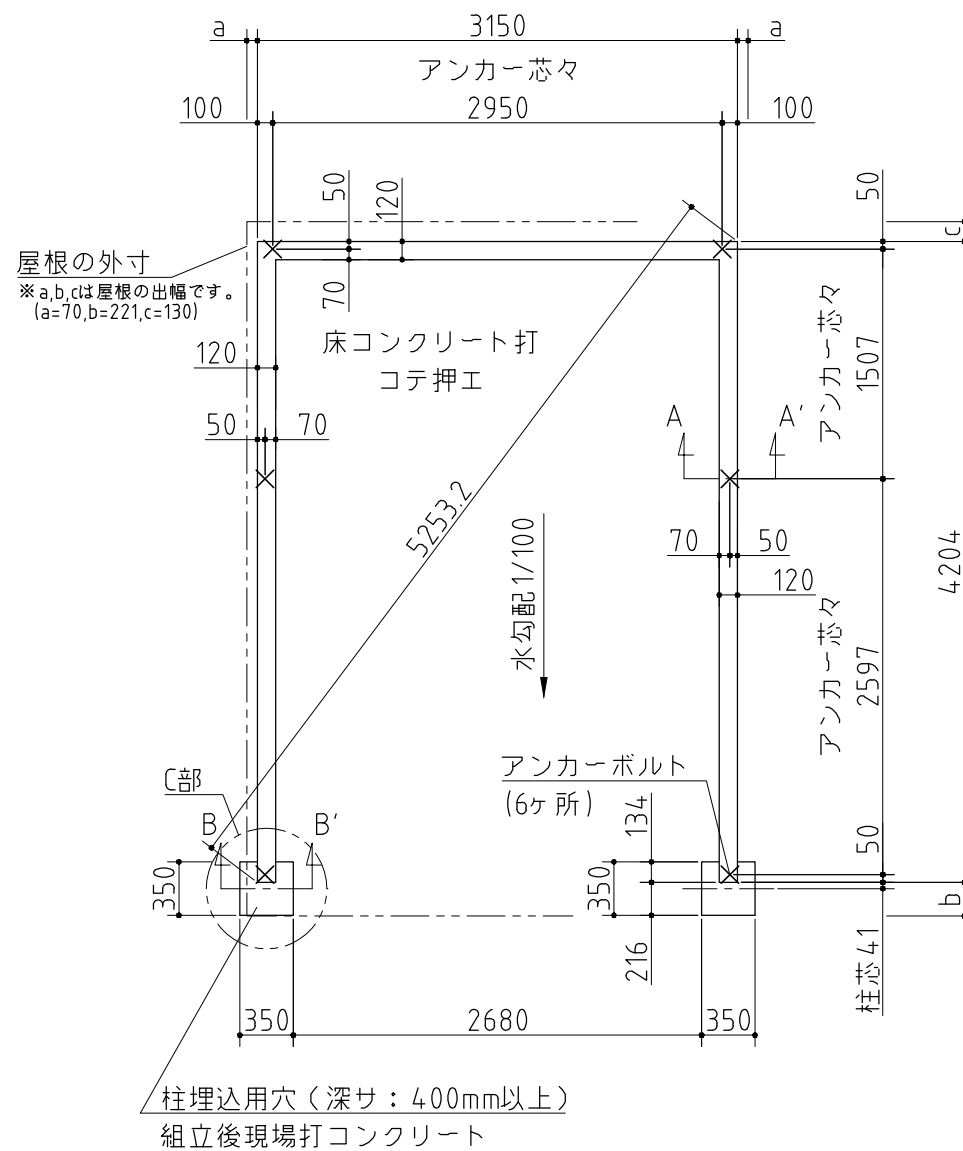
基礎詳細図 S=1/20
